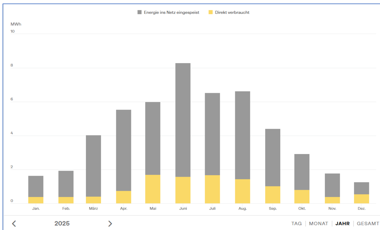
Bild 7.1: Darstellung des monatlichen Eigenverbrauches sowie Einspeisung im Betriebsjahr 2025
