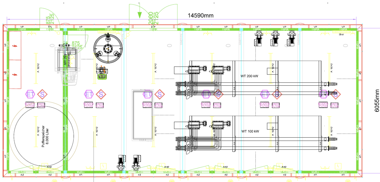
Abbildung 32: Raumbedarf zentrale Wärmeversorgung mit Rohrbündelwärmetauscher
