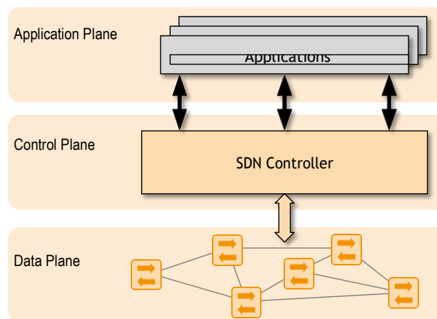
Abbildung 3. SDN Architektur
