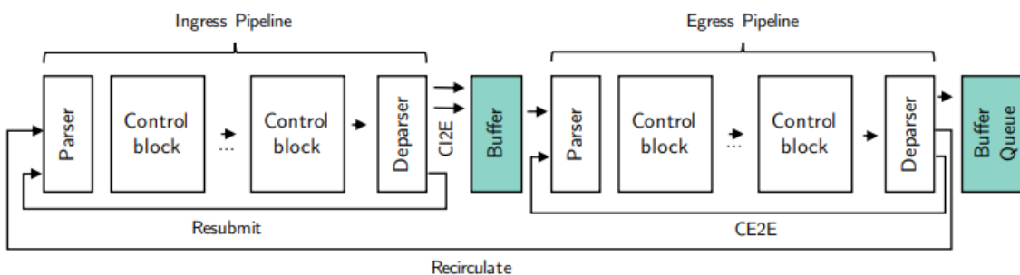
Abbildung 4. P4 Architektur
